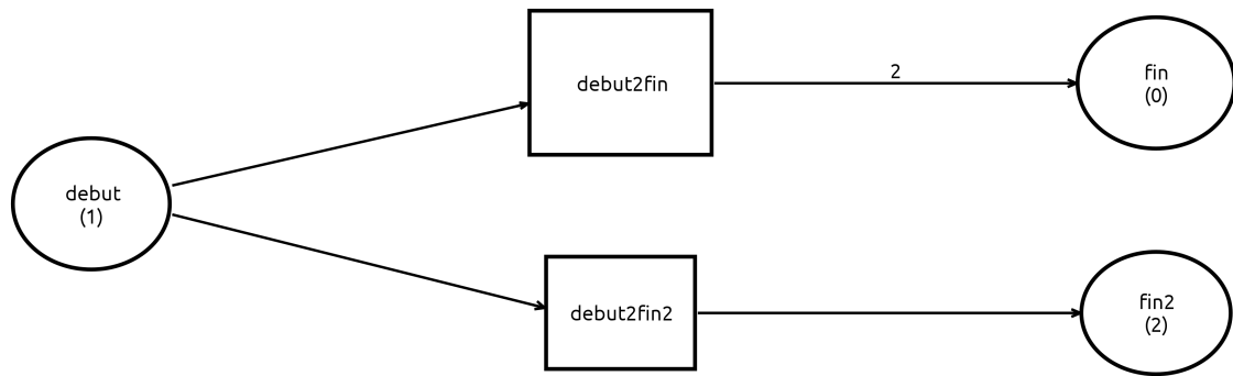
FIGURE 3 – Éditeur graphique d'un modèle petriNet
