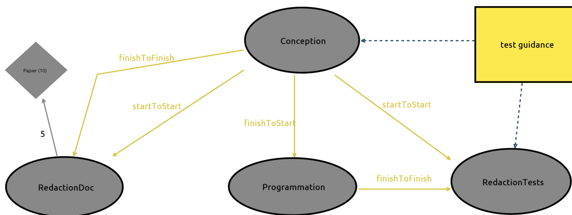
FIGURE 2 – Éditeur graphique d'un modèle simplePDL
