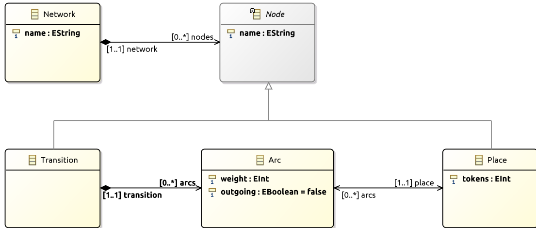
FIGURE 2 – Métamodèle petriNet complet
