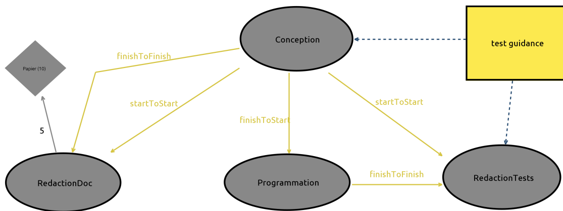
FIGURE 4 – Éditeur graphique d'un modèle simplePDL
