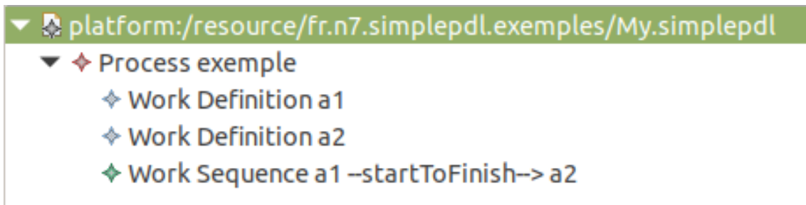
FIGURE 3 – Éditeur arborescent d'un modèle simplePDL
