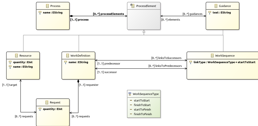
FIGURE 1 – Métamodèle simplePDL complet
