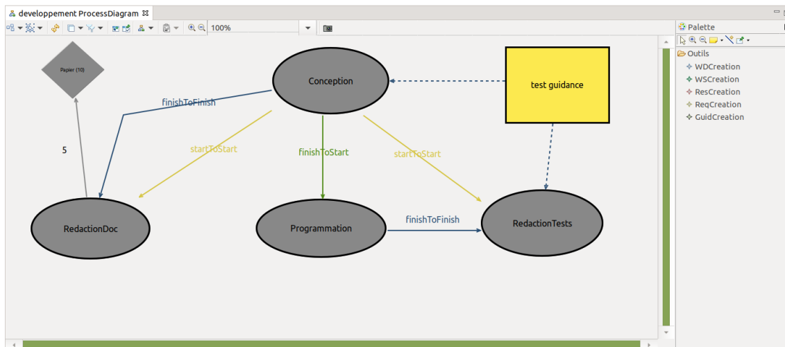
FIGURE 7 – Éditeur graphique d'un modèle simplePDL
